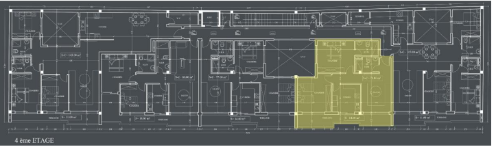
Plan Appartement-2 S-C : 78m 2
