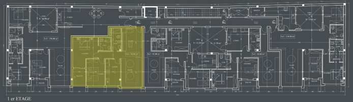
Plan Appartement-4 S-C : 98m²
