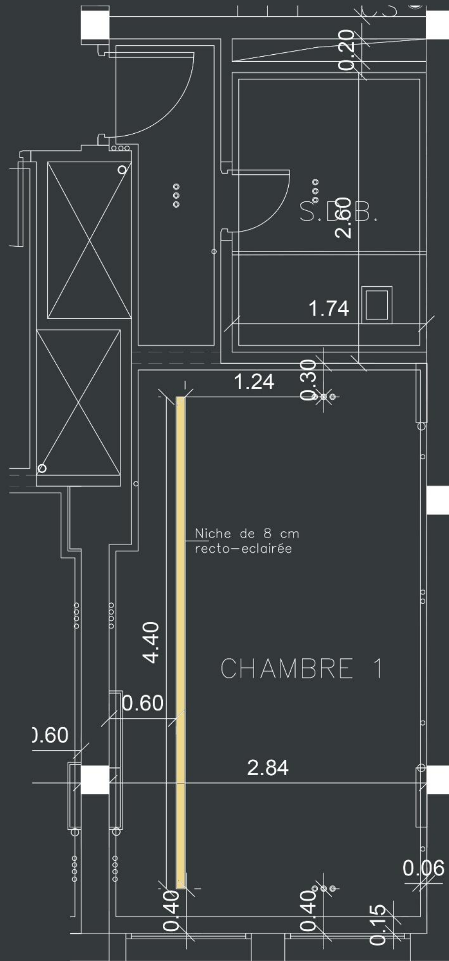
PLAN FAUX PLAFOND
