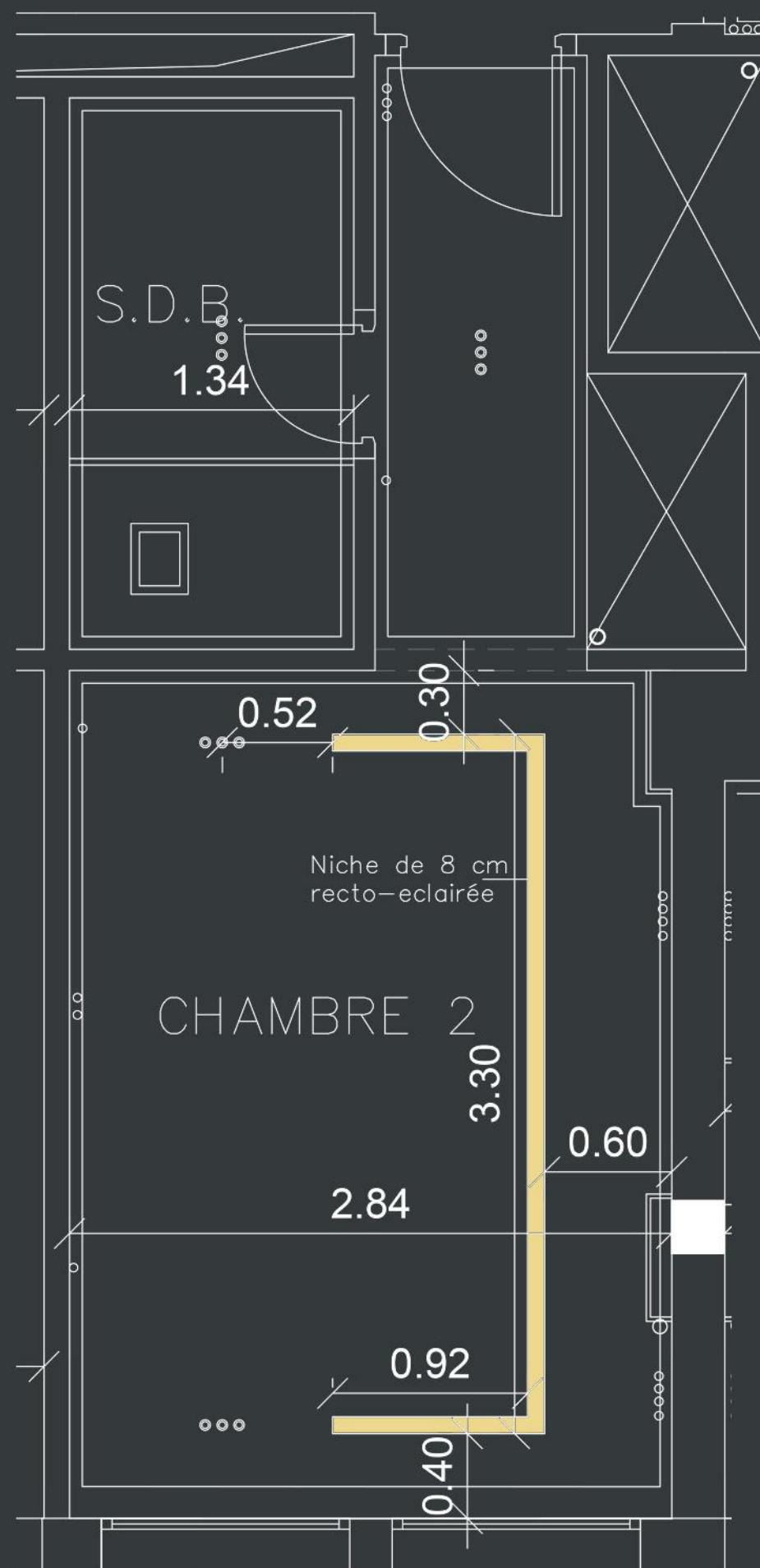
PLAN FAUX PLAFOND
