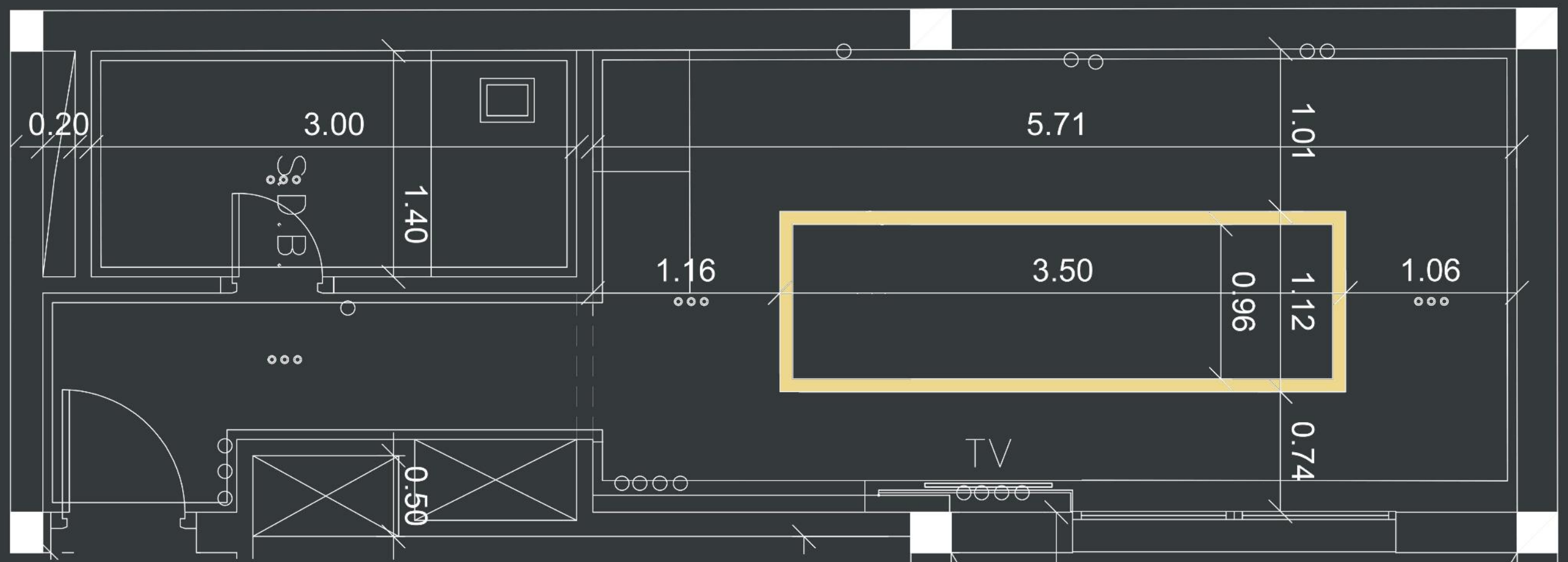
PLAN FAUX PLAFOND
